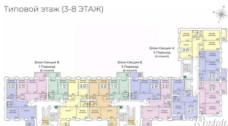
Типовой этаж (3-8 ЭТАЖ)
