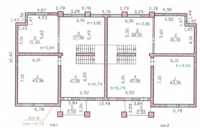
2 этаж
