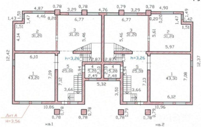
1 этаж
